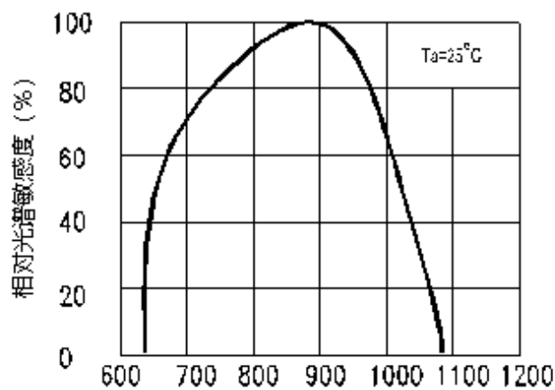
图一：光谱敏感度曲线
