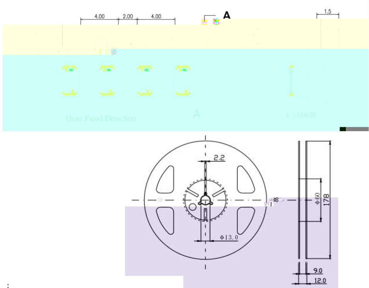
载带与圆盘尺寸
