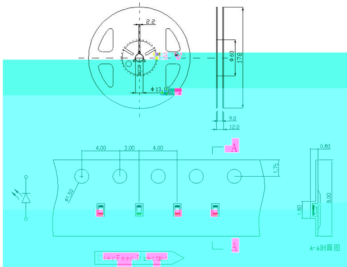
载带与圆盘尺寸
